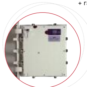
Verrouillage de la porte sur les 4 côtés par pènes tournants actifs/passifs chromés, nickelés, anti-sciage. Angle d'ouverture porte 200°.
